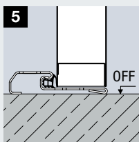
Упорная планка из нержавеющей стали, смонтирована в коробку
