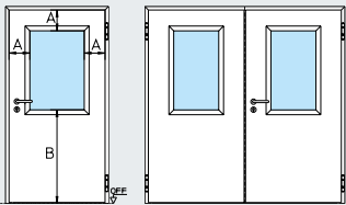
Остекление, рис. 2 Ширина кромки A: 270 мм Высота цоколя B: 965 мм
