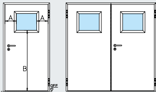
Остекление, рис. 0 Ширина кромки A: 270 мм Высота цоколя B: 1400 мм
