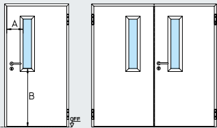
Остекление, рис. 1 Ширина кромки A: 270 мм Высота цоколя B: 965 мм
