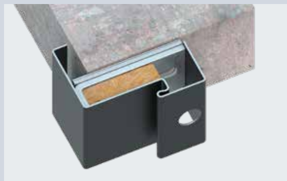
1. Установить и выровнять коробку в проеме
