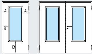
Остекление, рис. 3 Ширина кромки A: 270 мм Высота цоколя B: 500 мм
