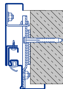
Охватывающая коробка (сост. из 2 частей) Зеркало дверной коробки 33 мм D тип 3
