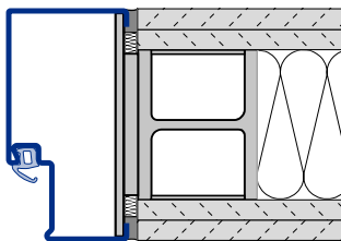
Блочная коробка, монтаж сваркой Е тип 1
