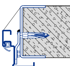
Угловая коробка Монтаж сваркой А тип 2 / А тип 3
