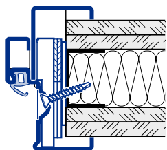
Универсальная угловая коробка с дополнительной коробкой Vario B53 Диагональное крепление С тип 1
