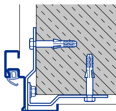
Угловая коробка Монтаж через угол стены А тип 2 / А тип 3
