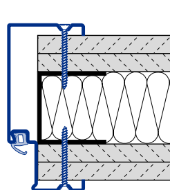
Охватывающая коробка B73 для каркасных стен Монтаж на винтовых соединениях С тип 4
